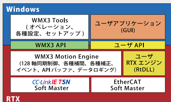
ソフトウェア構成図
